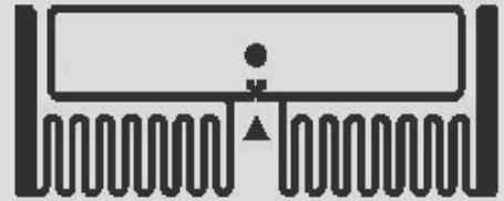
天线示意图
